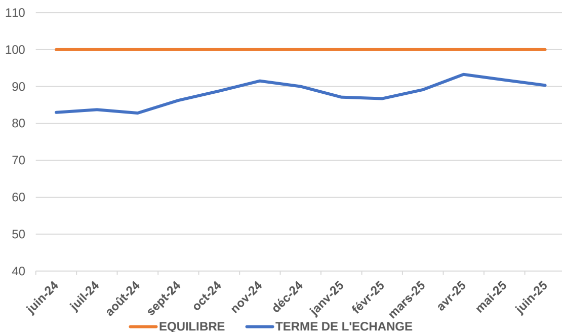
Graphique 2 : évolution des termes de l'échange
